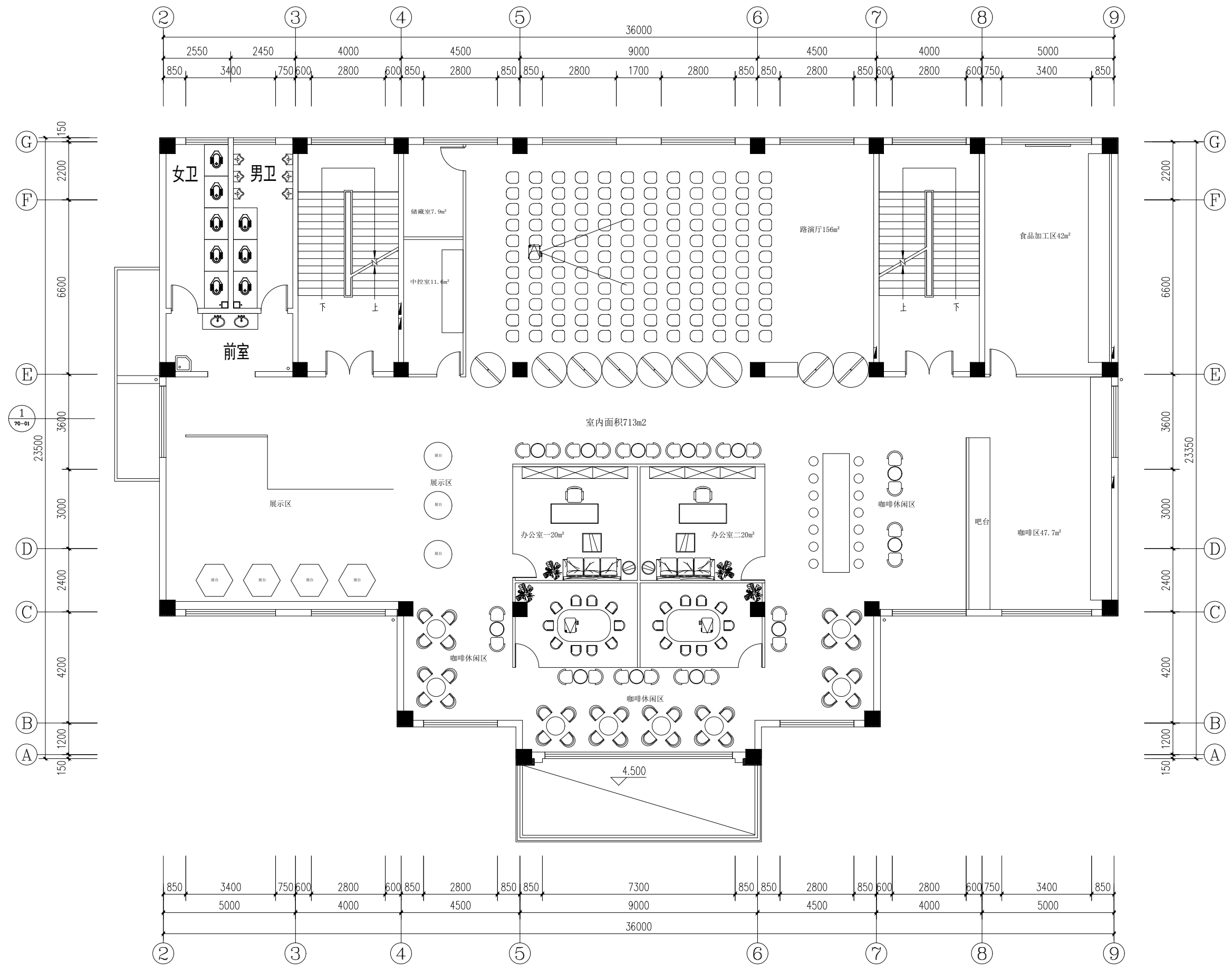
二层平面布置图 1:150
